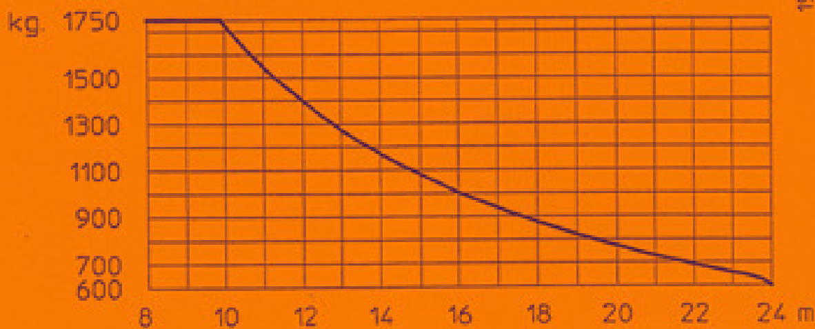
LASTDIAGRAMM mit horizontalem Ausleger
