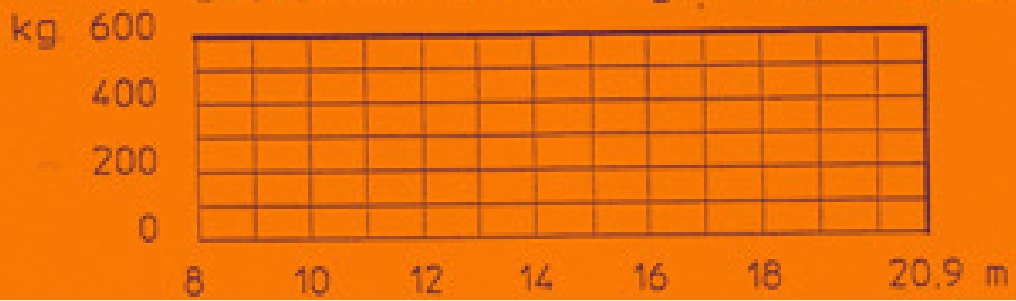
LASTDIAGRAMM mit stielgestelltem Ausleger
