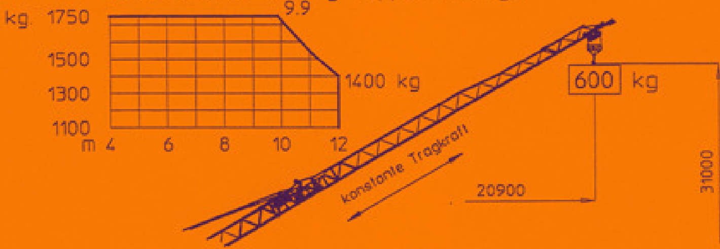
LASTDIAGRAMM mit eingeklapptem Ausleger
